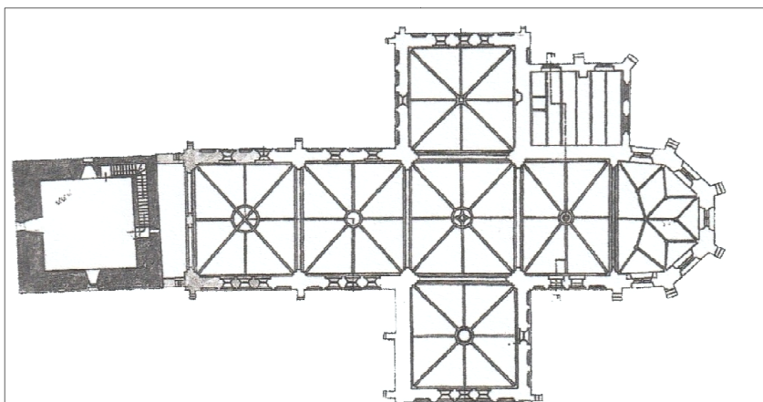
Stedum, Bartholomeüskerk, plan eerste etage toren. Situatie voor inbouw klokkenstoel.
