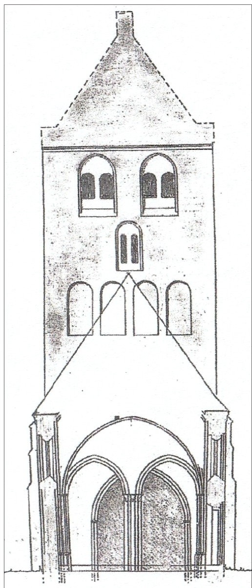
Stedum, Bartholomeüskerk, doorsnede over het schip. Situatie voor inbouw klokkenstoel.
